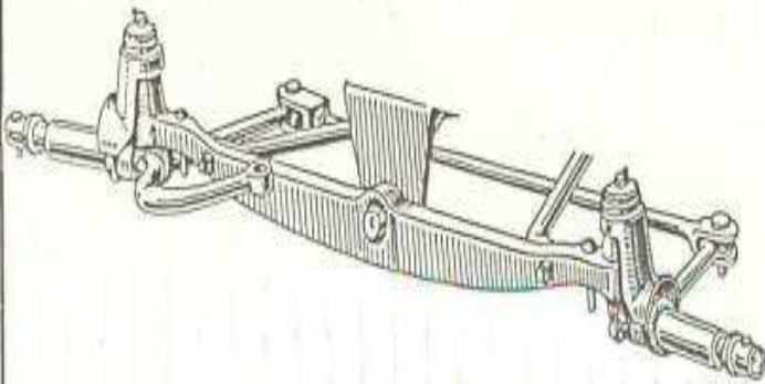
Vorderachse mit Nabe gefedert / ungefedert
