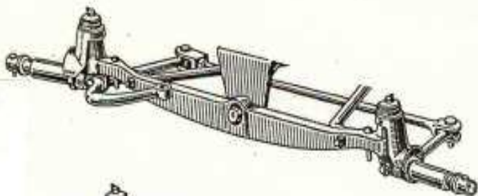
Vorderachse mit Naben
